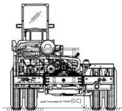
Tampak Belakang
