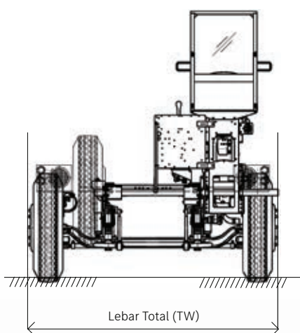
Tampak Depan
